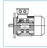
IM B35 IM 2001
